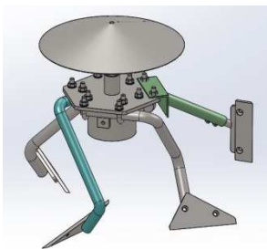
B140-Mischwerkzeug
