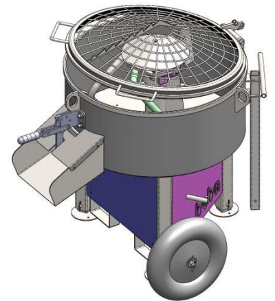
Verkleidung-Hardox
